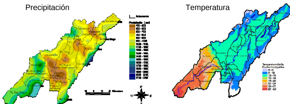
Figura 3-1 Temperatura y Precipitación en la cuenca
